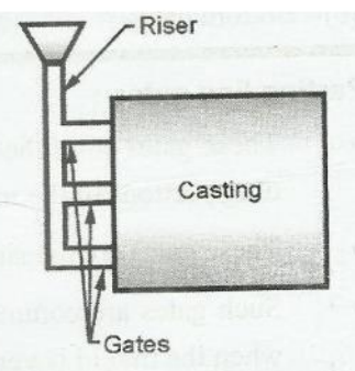
Fig. 1.37 Side gate
