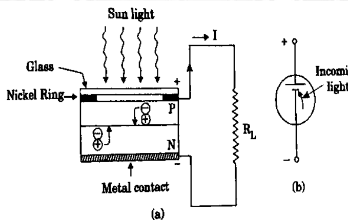
Fig 4.4.1 Solar cell
